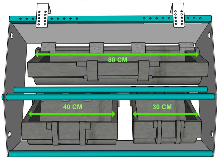
Exemple de configuration de positionnement de godets
